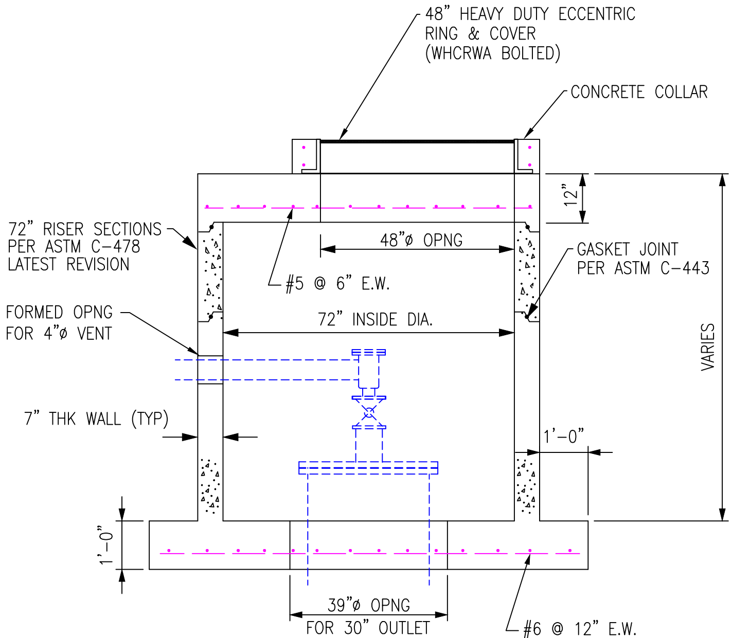
MANHOLE SECTION
