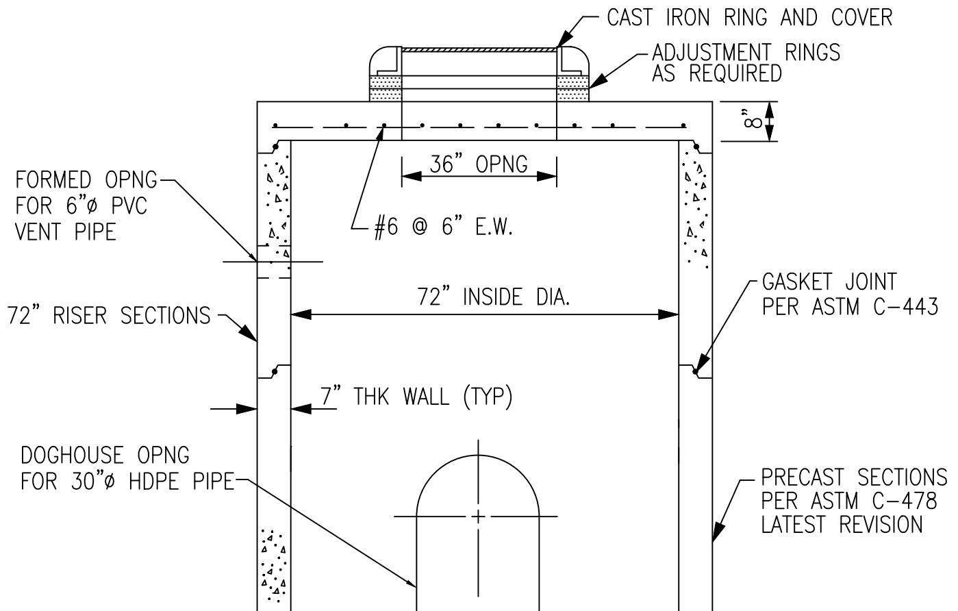
MANHOLE SECTION
