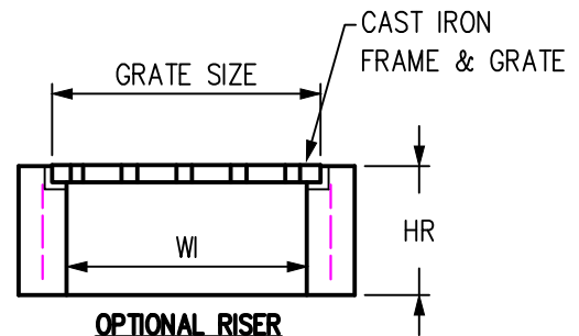
OPTIONAL RISER
